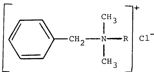
FIG. 1. Benzalkonium Chloride.
